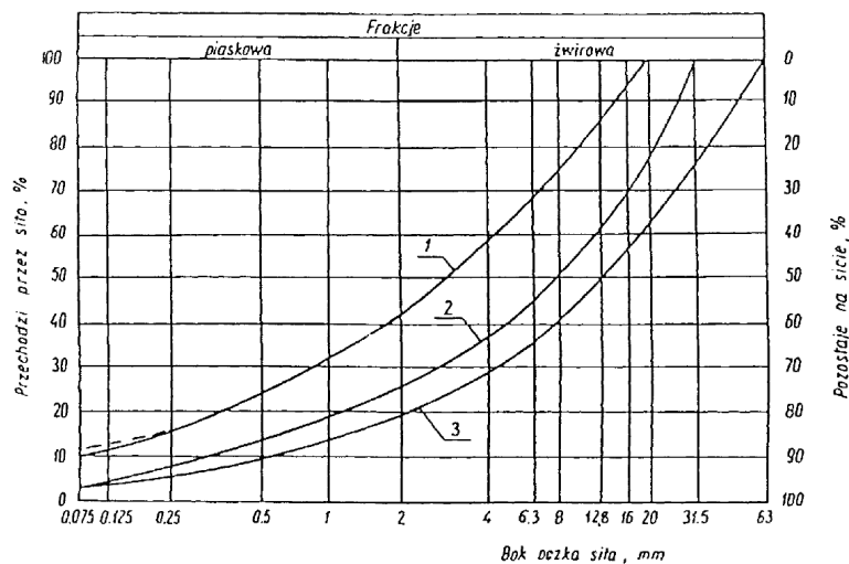
Rysunek 1. Pole dobrego uziarnienia kruszyw przeznaczonych na podbudowę wykonywaną metodą stabilizacji mechanicznej
